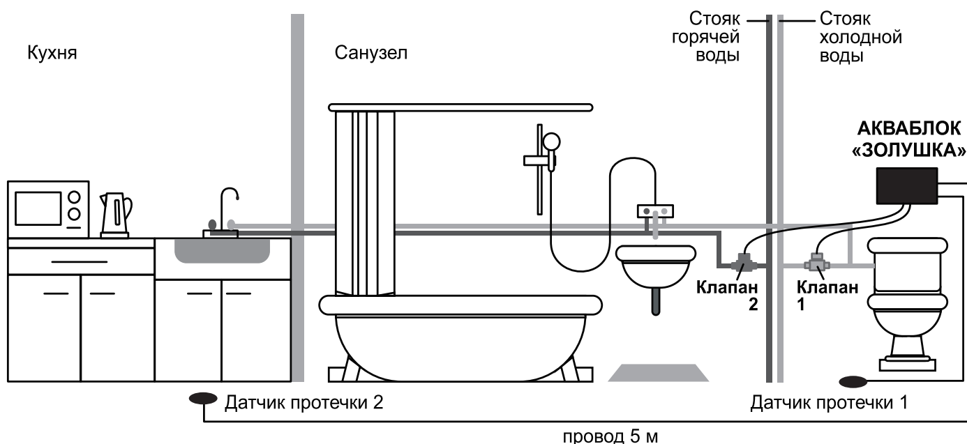
Рис.3 «Пример установки системы»
